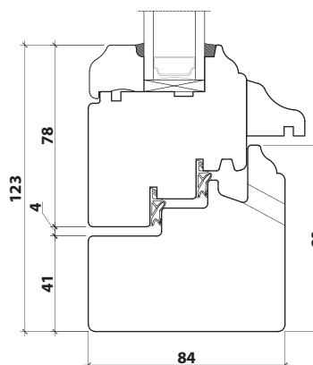
PARTIE BASSE
