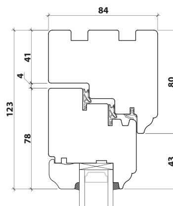
PARTIE HAUTE
