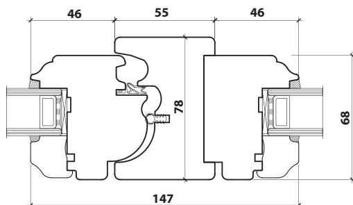
MENEAU MOBILE
