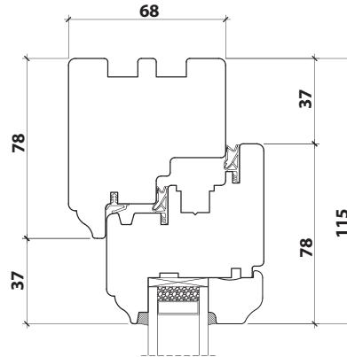
PARTIE HAUTE
