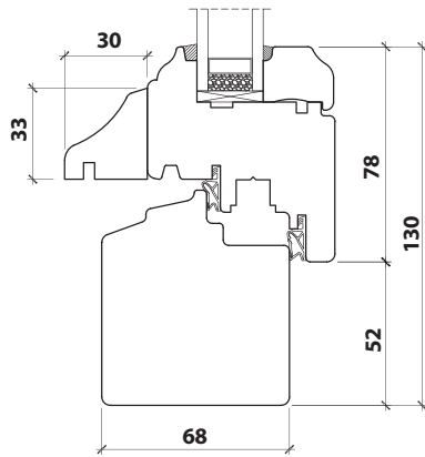
PARTIE BASSE
