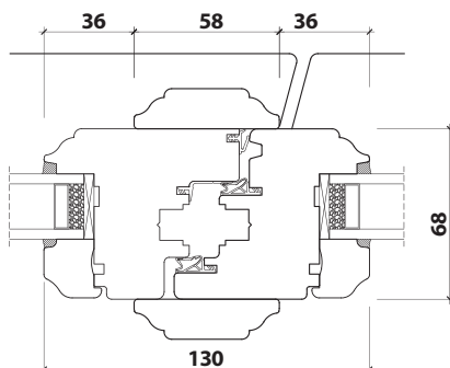
POIGNÉE CENTRÉE
